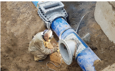
강관 분기 시공
