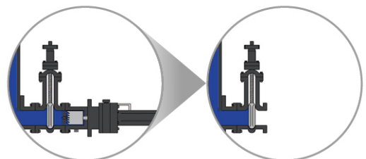
⑤ 시공완료(제수밸브 닫고 천공기 탈거)
